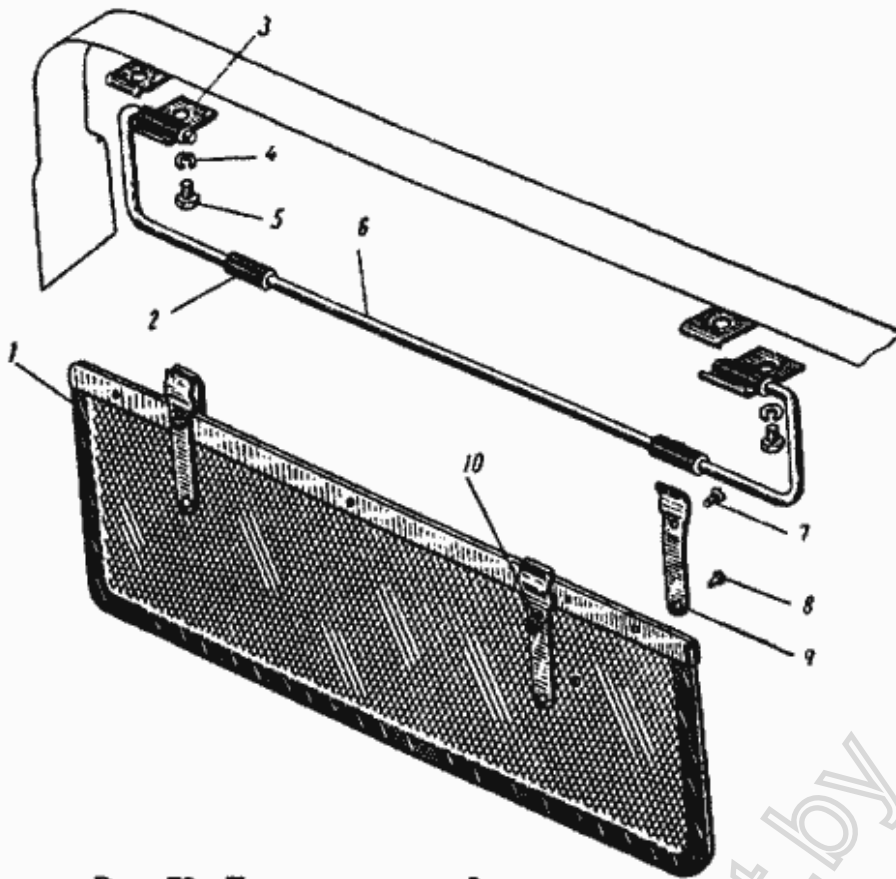
Рис. 72. Противосолнечный козырек
